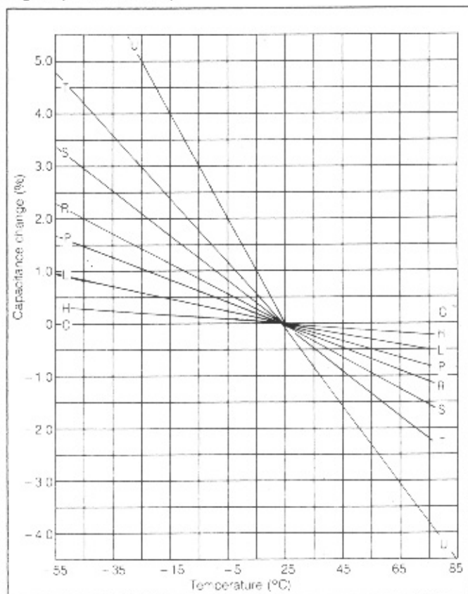
Fig. 1 (T.C. PPM/°C)
